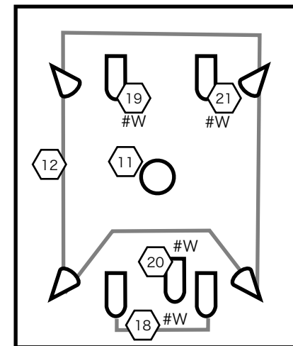
LIVEHOUSE 箱船 照明図 2023.3.31
